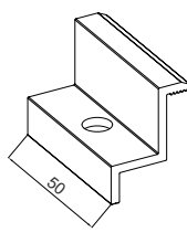
Klema końcowa 90432/P01
