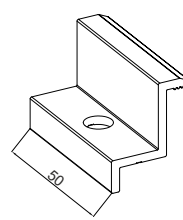
Klema końcowa 90457/P01
